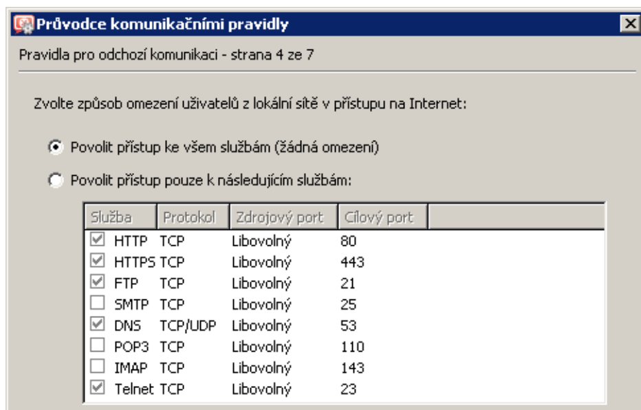
Obrázek 23.55 Pobočka Brno — přístup z lokální sítě do Internetu bez omezení
