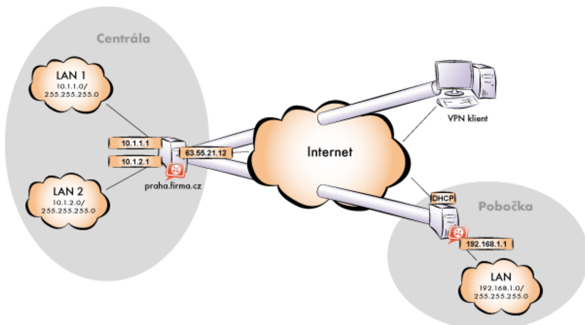
Obrázek 23.12 Příklad — propojení centrály a pobočky firmy VPN tunelem s možností připojení VPN klientů
