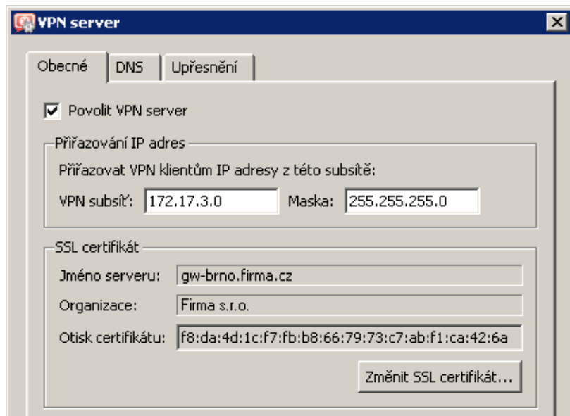
Obrázek 23.59 Pobočka Brno — konfigurace VPN serveru
