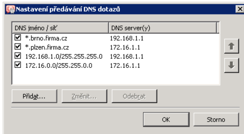
Obrázek 23.36 Centrála — nastavení předávání DNS dotazů
