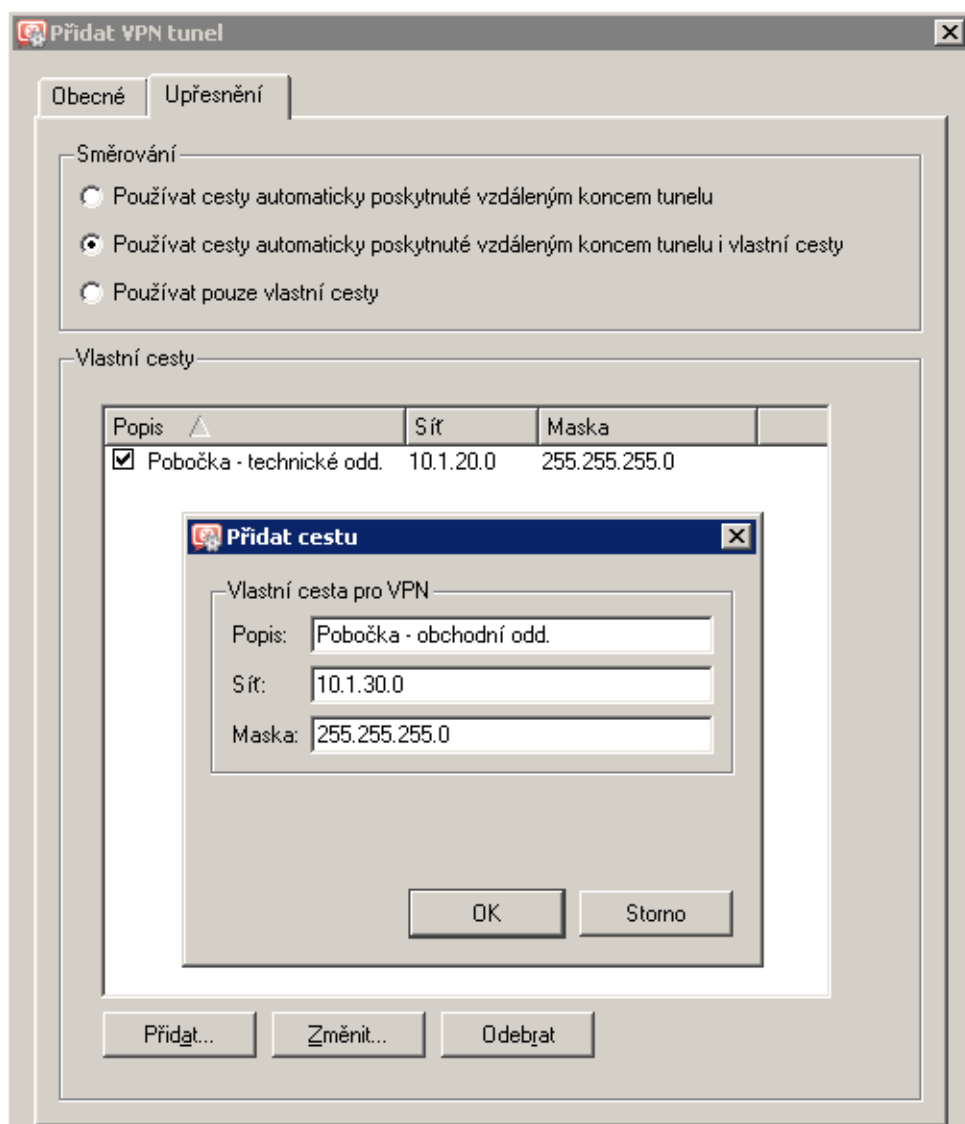
Obrázek 23.9 Nastavení směrování pro VPN tunel
