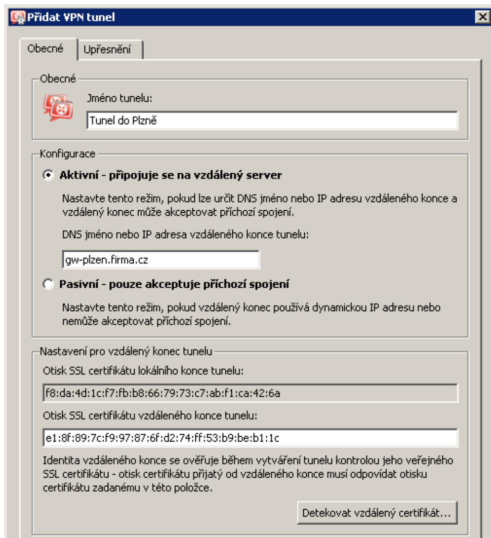
Obrázek 23.62 Pobočka Brno — definice VPN tunelu do pobočky Plzeň
