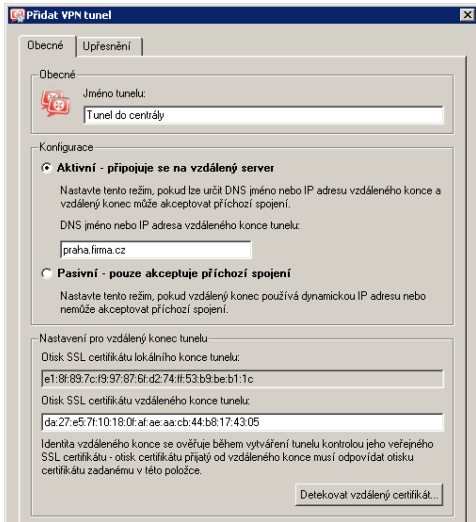
Obrázek 23.29 Pobočka — definice VPN tunelu do centrály
