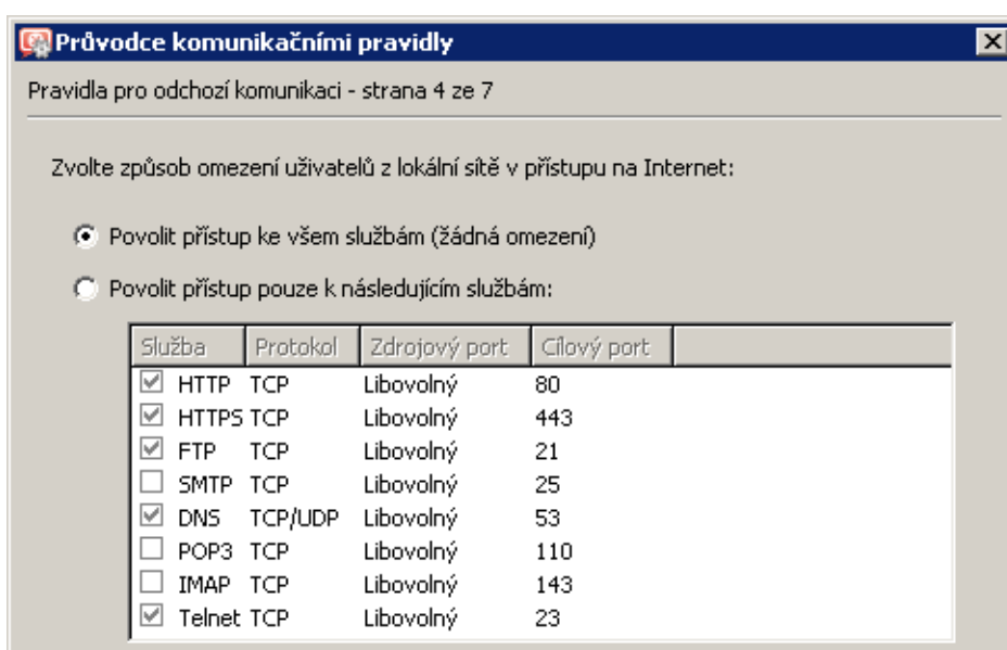
Obrázek 23.44 Pobočka Plzeň — přístup z lokální sítě do Internetu bez omezení
