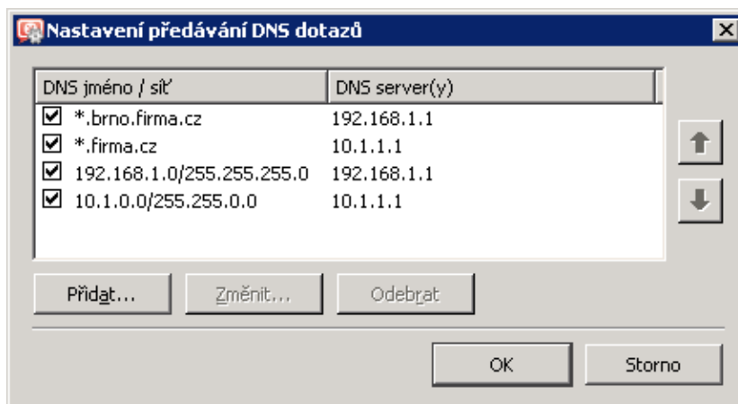
Obrázek 23.48 Pobočka Plzeň — nastavení předávání DNS dotazů
